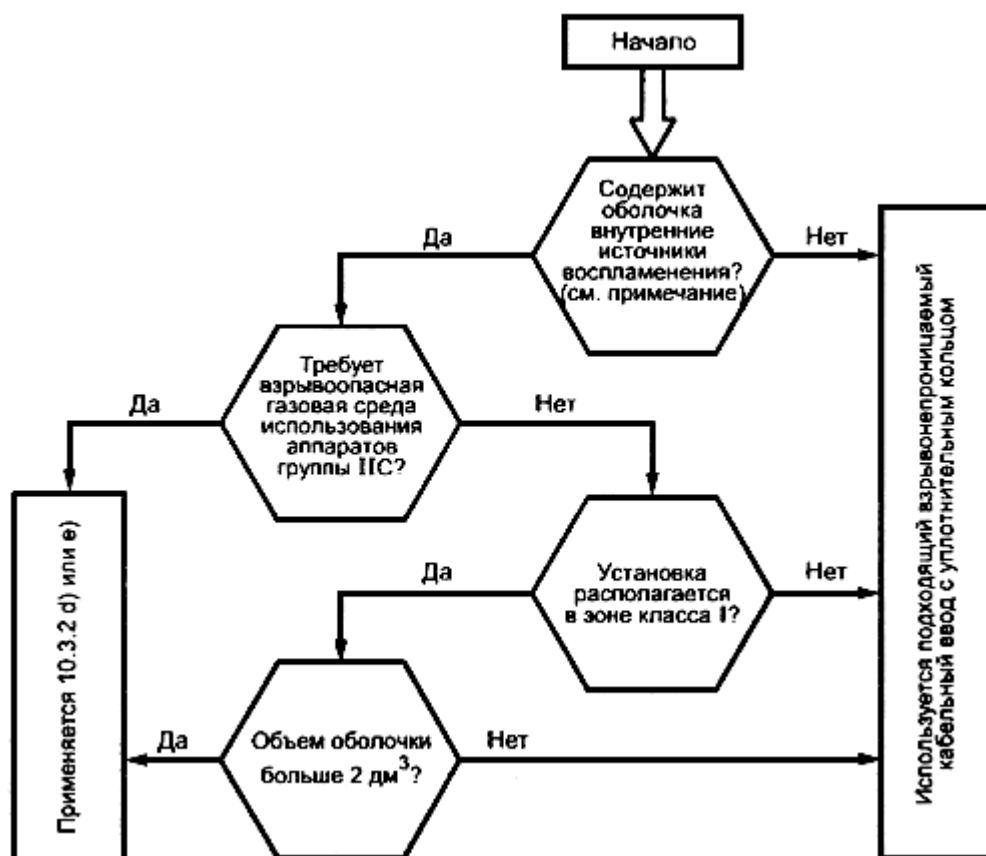
Рисунок 1 - Схема выбора кабельного ввода во взрывонепроницаемые оболочки
